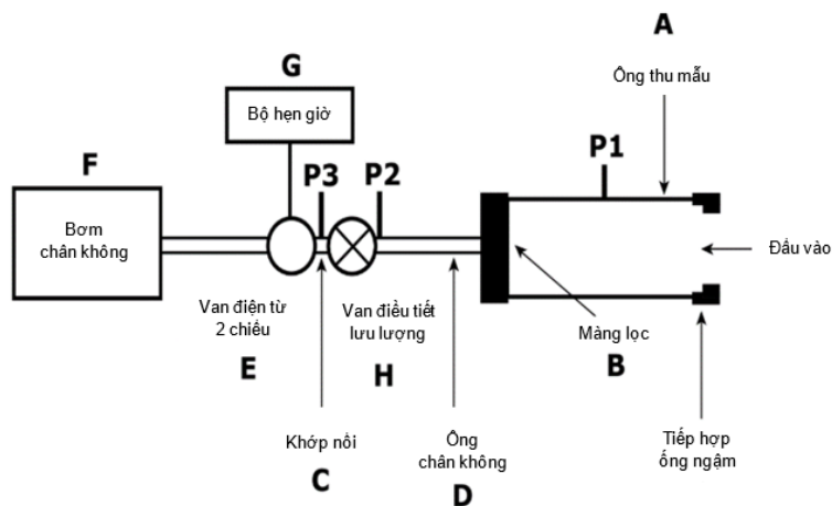
Hình 1.17.2 - Thiết bị để đánh giá Độ đồng đều liều phân phối của thuốc bột hít
